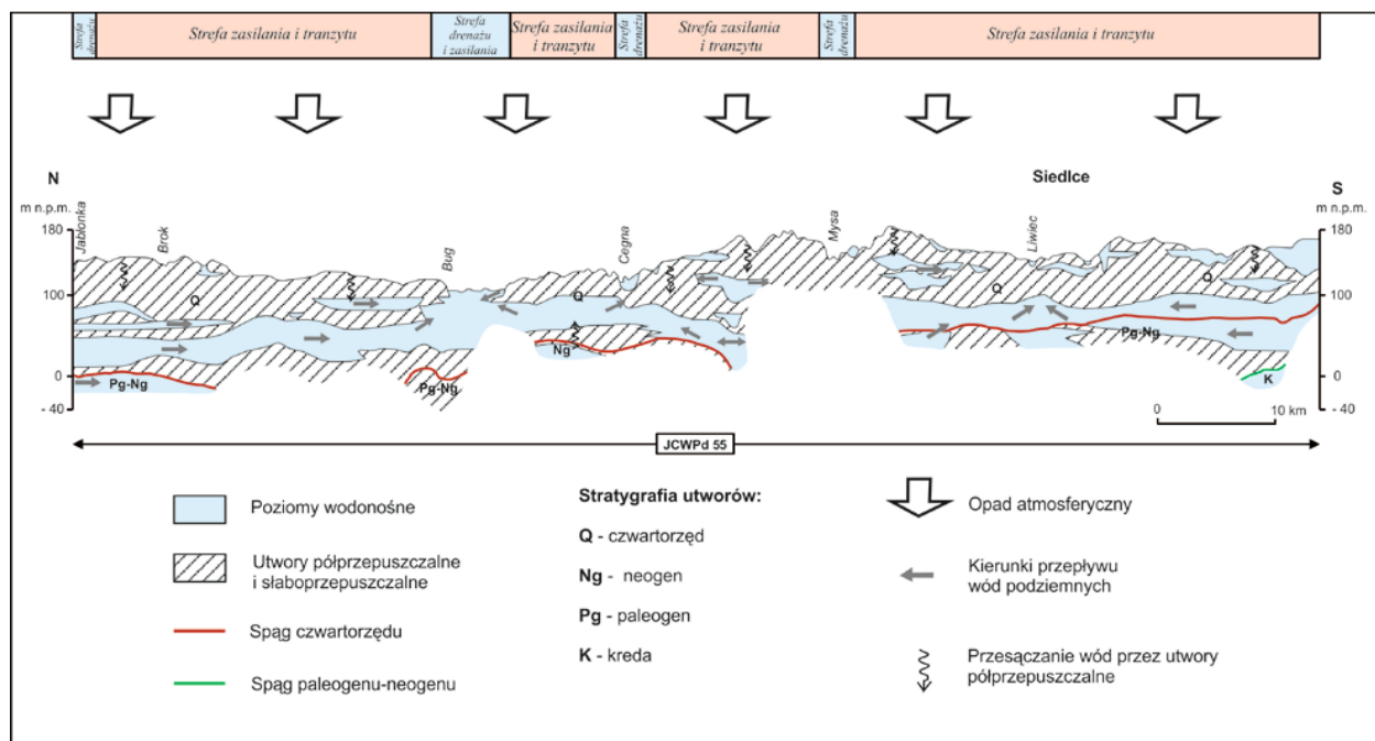
Ryc. 10. Schemat przepływu wód podziemnych w granicach JCWPd 55.
