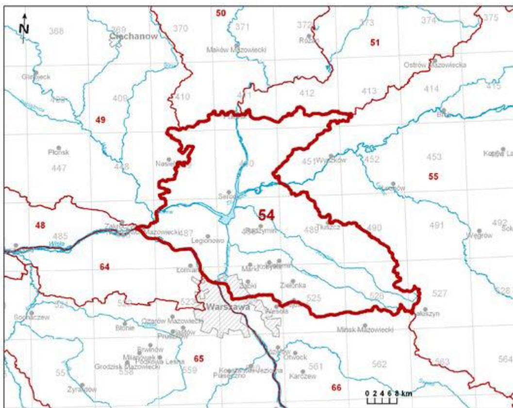
Ryc. 7. Zasięg JCWPd 54.
