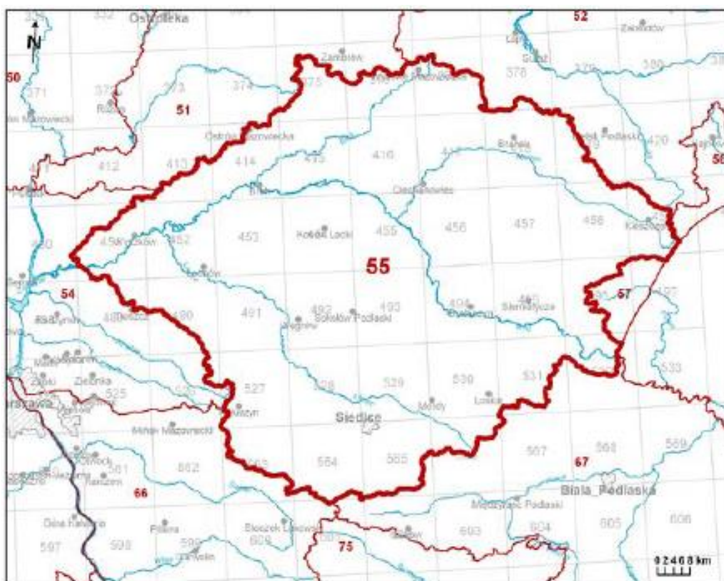
Ryc. 9. Zasięg JCWPd 55.
