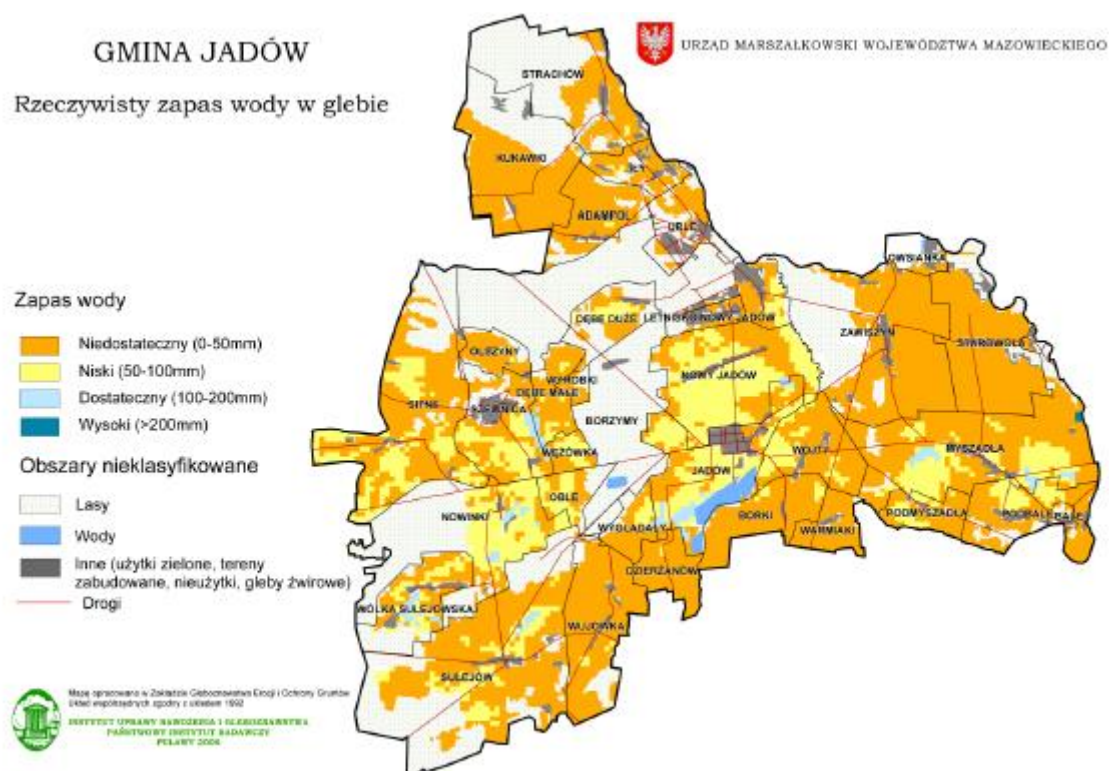
Ryc. 14. Wycinek mapy rzeczywistego zapasu wody w glebie powiatu wołomińskiego ( Prognoza oddziaływania na środowisko Studium uwarunkowań i kierunków zagospodarowania przestrzennego gminy Jadów, Warszawa, 2016 )
