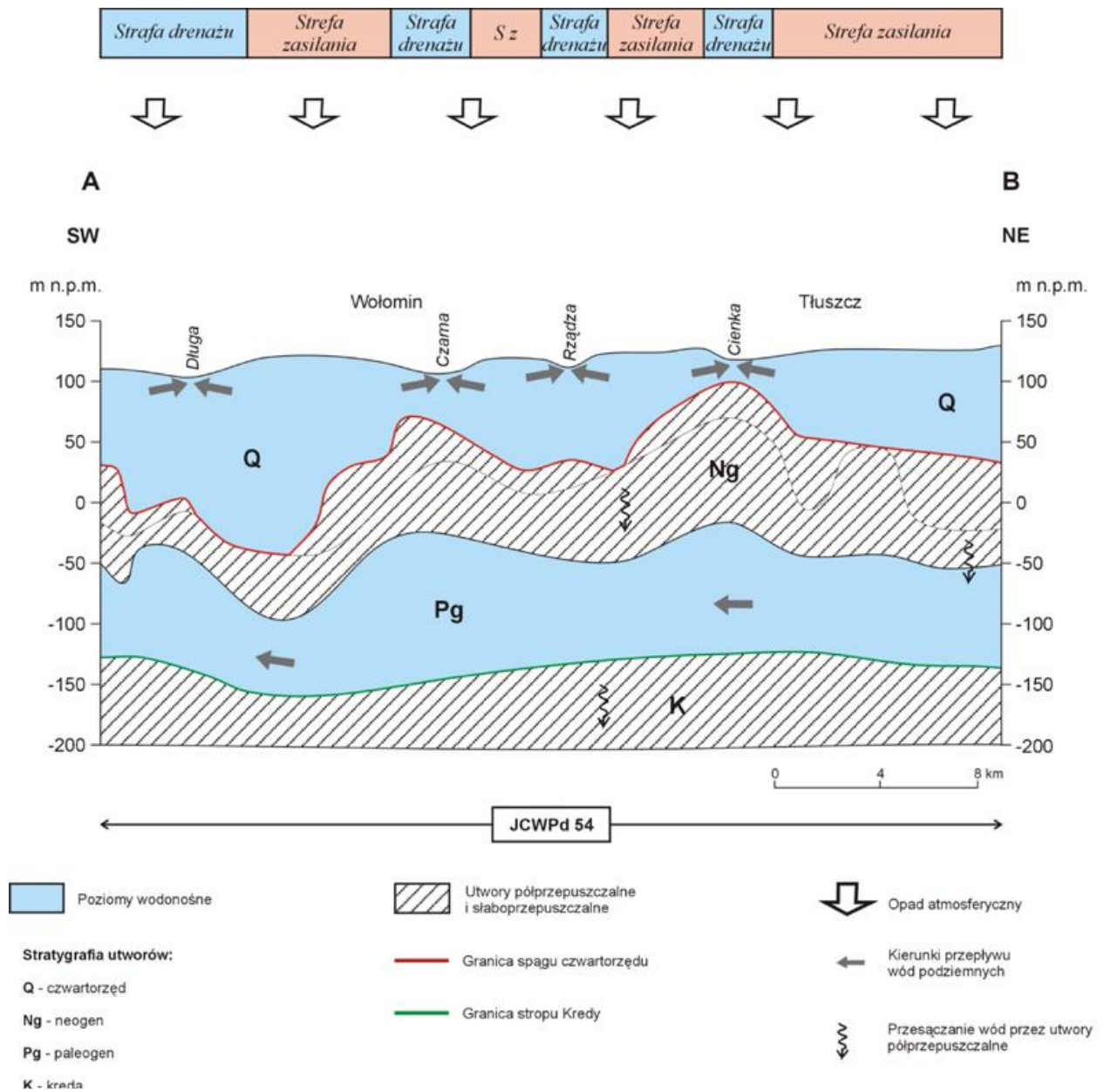
Ryc. 8. Schemat przepływu wód podziemnych w granicach JCWPd 54.
